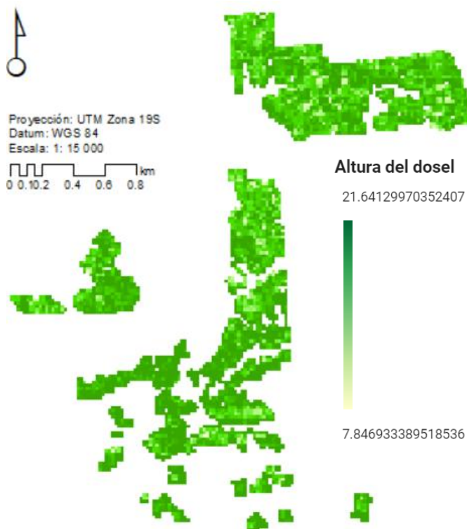
Figura 9. Modelo de altura del dosel obtenido mediante Random Forest, combinando GEDI 2A con Sentinel-1, -2 y datos de elevación digital.
